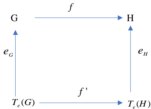
Figura N° 10 Conmutatividad entre Homomorfismos de grupos de Lie con los inducidos de álgebras de Lie.
